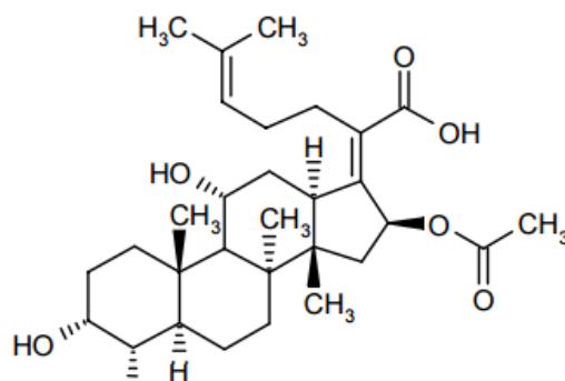
Figura 1: Fórmula Molecular do Ácido Fusídico.
