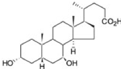
Figura 1: Formula Molecular do Ácido Ursodesoxicólico.
