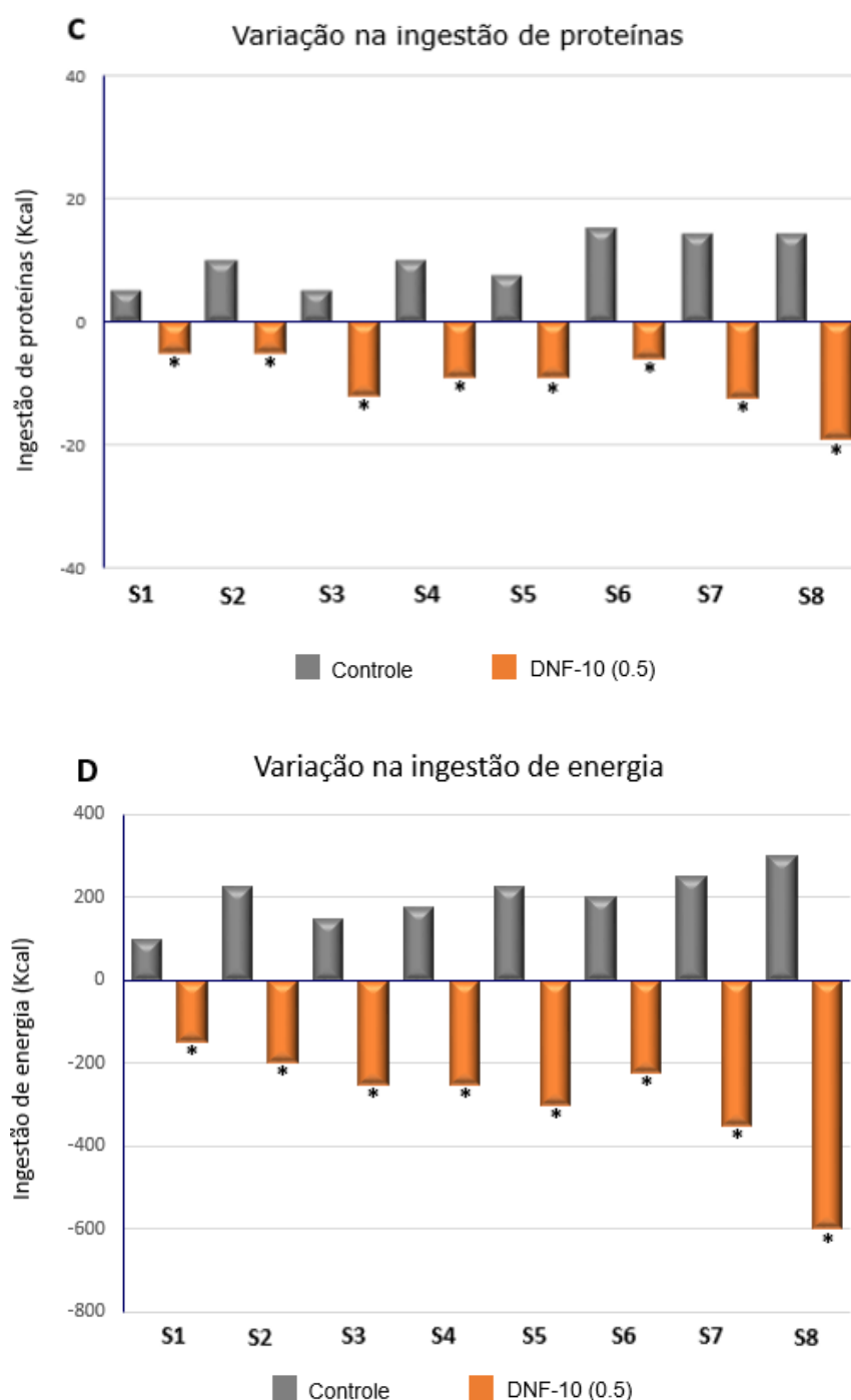
Gráfico 4. Variações na ingestão de carboidratos ( A ), lipídios ( B ) e proteínas ( C ) durante 8 semanas com DNF-10/500 . A redução na ingestão calórica é significativa a partir da primeira semana de suplementação com DNF-10 comparado ao grupo controle. Após 8 semanas, os indivíduos diminuíram sua ingestão calórica diária em 600 kcal, enquanto que no grupo controle a ingestão calórica diária aumentou em 276 kcal. Essa redução veio principalmente de carboidratos, mas a redução na ingestão de lipídios e proteínas também contribuiu ( D ).
