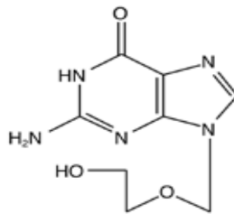
Figura 1. Estrutura química do Aciclovir (9-(2-Hydroxyethoxymethyl)guanine).
